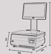
DIMENSÕES (MM)
